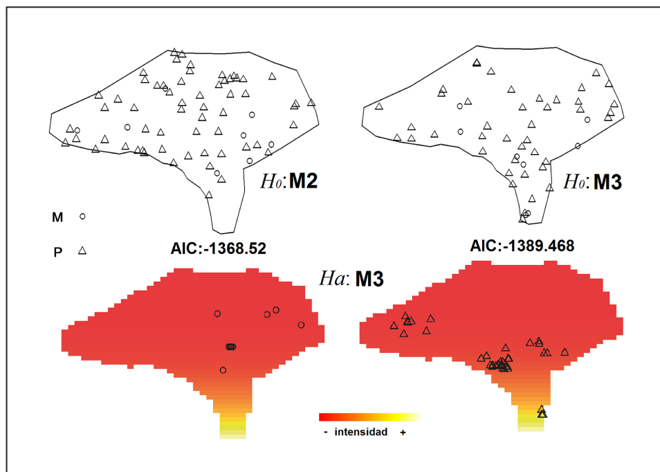
Figura 5. H0 M2: simulación del patrón esperado bajo modelo aleatorio en relación a las categorías artefactuales y valor de AIC del modelo ajustado. H0 M3: simulación del patrón esperado bajo modelo aleatorio en relación a las categorías artefactuales y un gradiente de densidad N-S y valor de ajuste del modelo. HaM3: Gradiente de densidad esperada (predicha) por el modelo para morteros (izquierda) y pesas (derecha). M: morteros. P: pesas.
